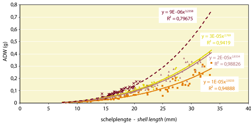
Figuur 8. Vleesgewicht ten opzichte van schelpenlengte voor vier soorten tweekleppigen tijdens de WOT benthos surveys in 2016. Ash-free dry weights of flesh as a function of shell length in four species of bivalves (2016 benthos survey).
