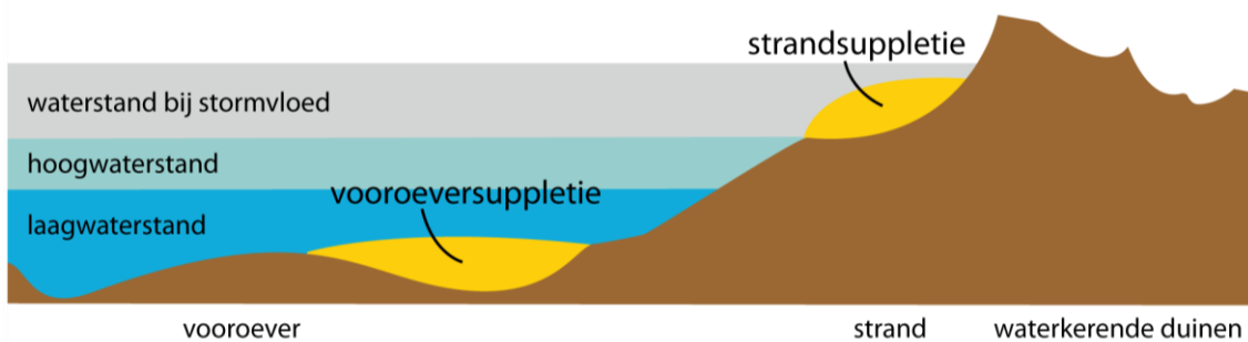
Figuur 6.1 Vooroeversuppletie en strandsuppletie
