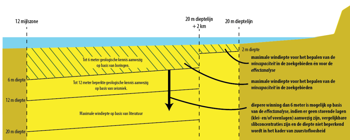
Figuur 8.1 Schematische weergave plangebied en windieptes
