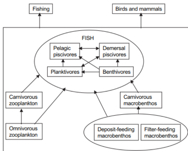
Figuur 10.3 Voedselketenrelaties voor vissen (Heath, 2005)
